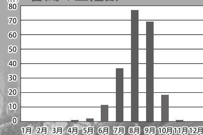
(件) 台風の上陸数(1951年~2023年)
