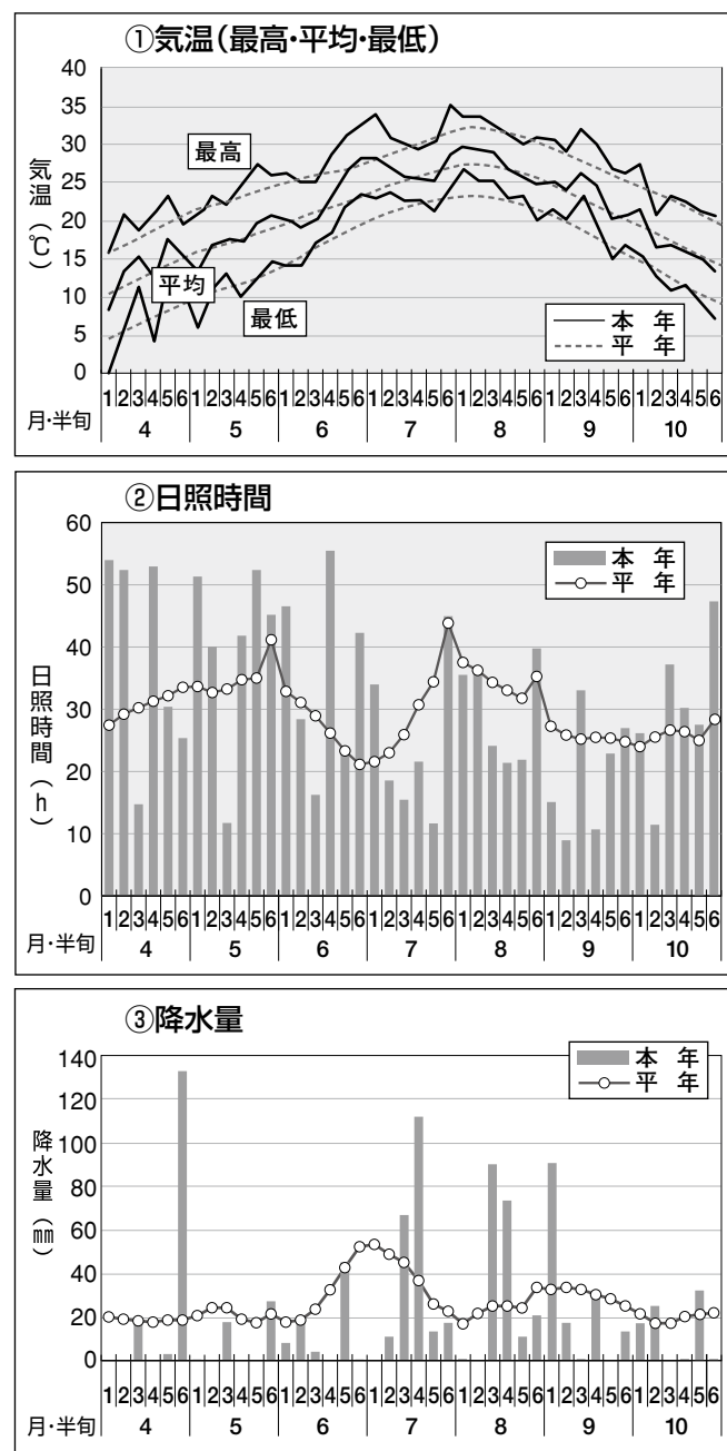
図1 令和4年気象（出雲市）
