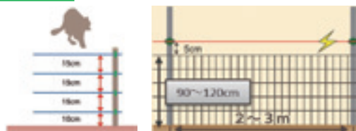
アナグマ対策の電柵と複合柵
