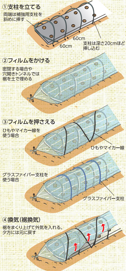
図 トンネルの作り方
